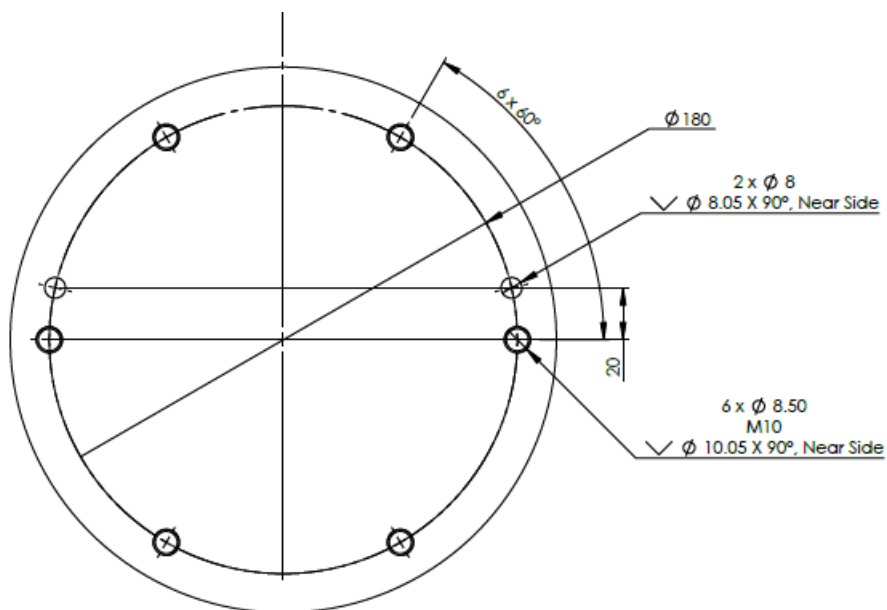
1.1: Undersiden av robotbasen
